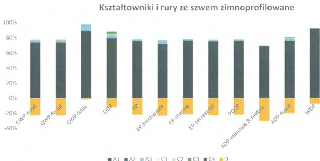
Rysunek 6 Udziały modułów cyklu życia na główne kategorie wpływów – kształtowniki i rury ze szwem zimnoprofilowane.
